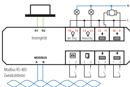
Beispiel: Funktionsbelegung für Option 2 beim Modbus-Hotelregler.
