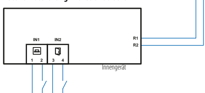
Beispiel: Funktionsbelegung für neue Einzel-Hotelfernbedienung mit Touch-Screen.
